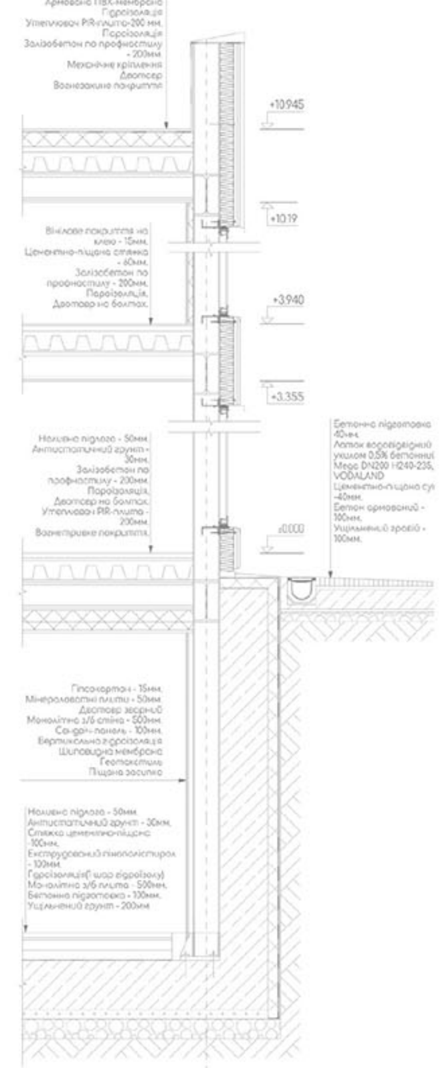
Детальний розріз по стіні М 1:20
