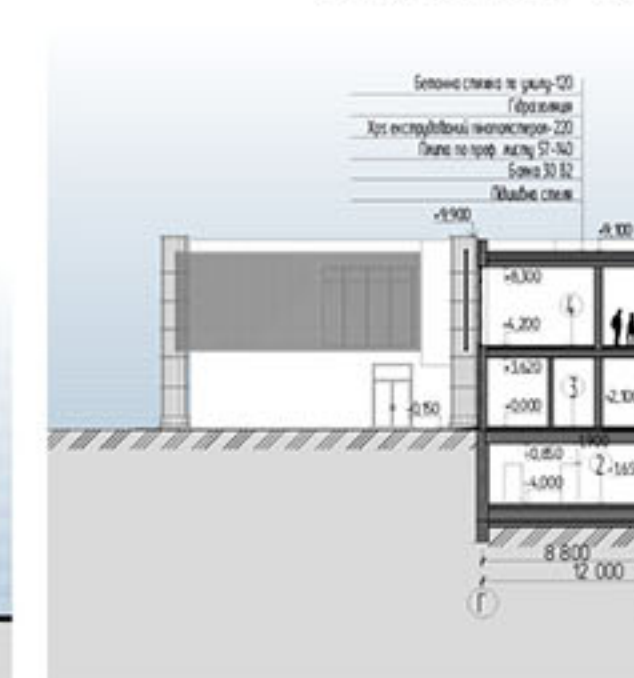
Розріз 2-2 М 1:200
