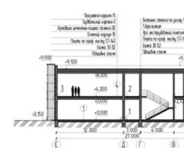
Розріз 3-3 М 1:200
