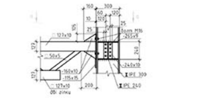
Вузол А
