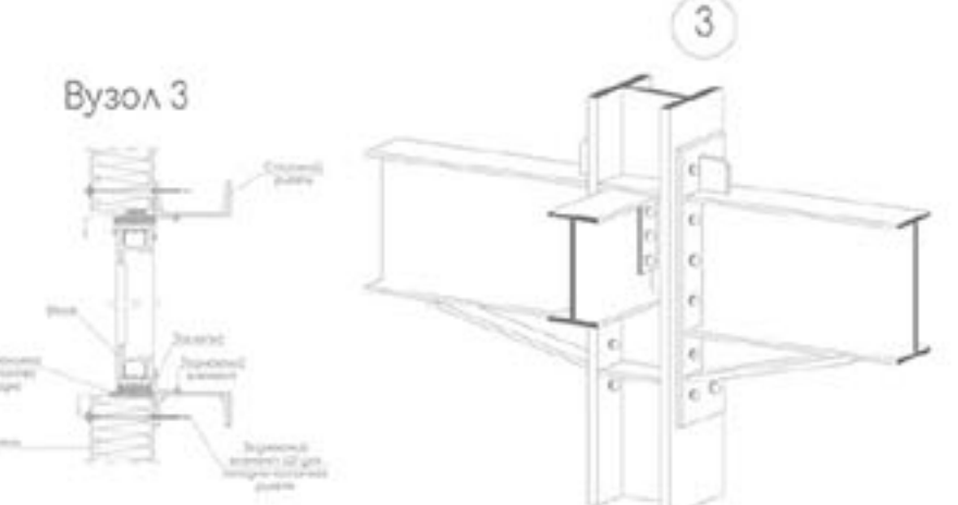
Вузол 3
