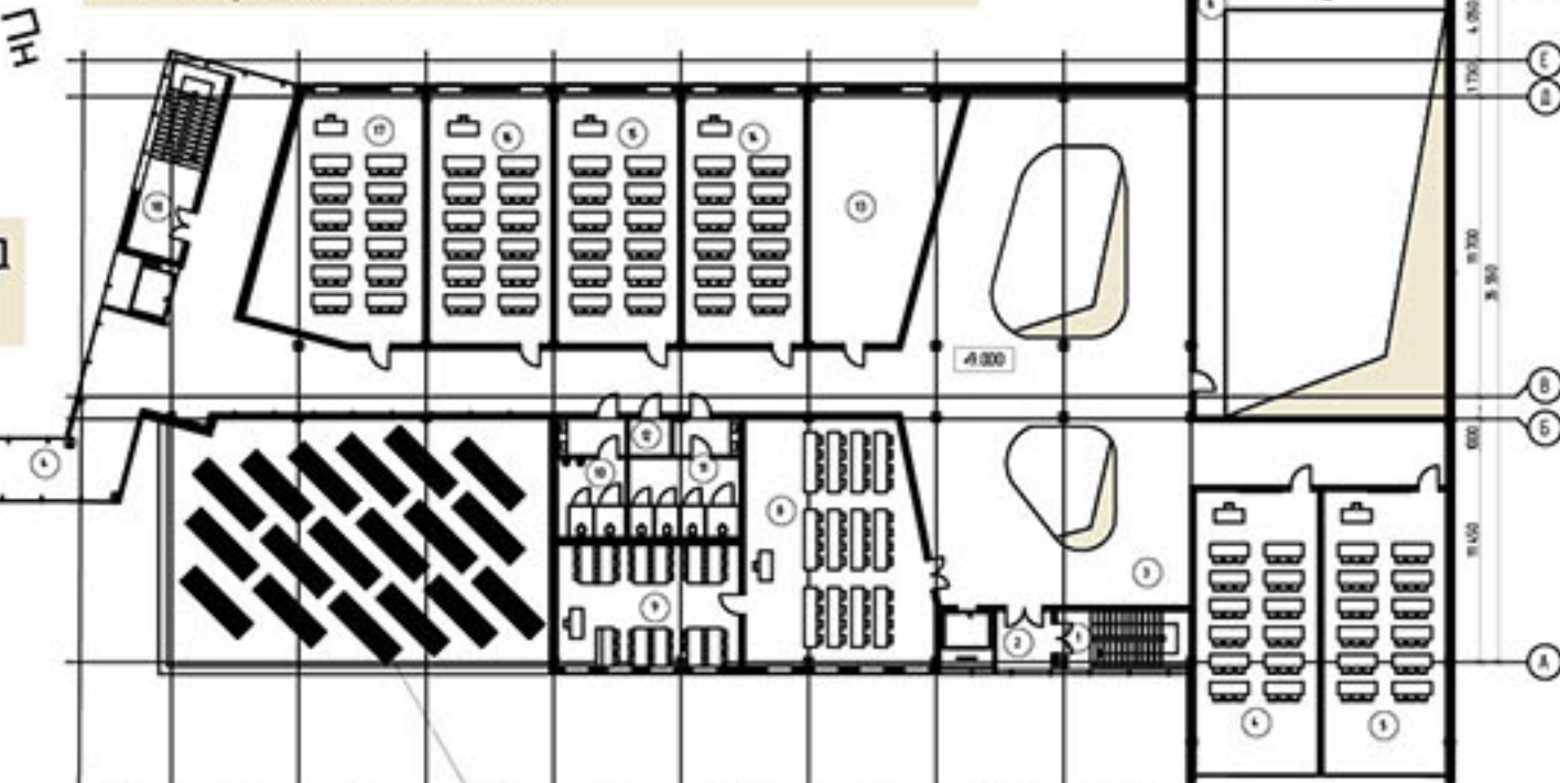
План третього поверху корпусу №7 на відмітці +9.000 М1:200
