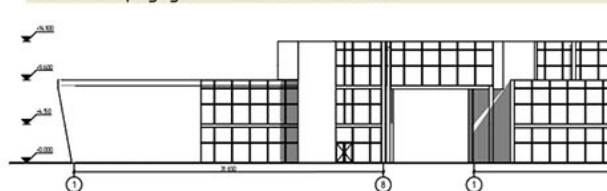
Фасад корпусу №11 в осях 1-8 М1:200
