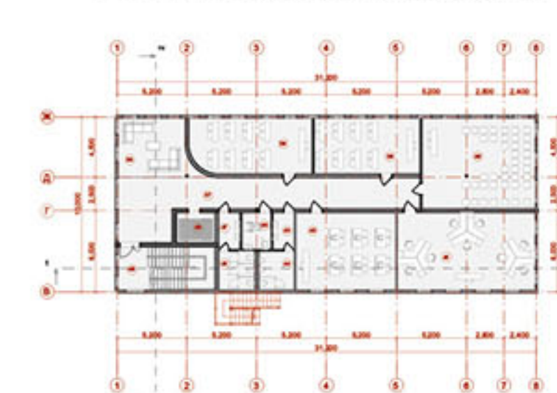
План на відмітці +3,000 М1:200
