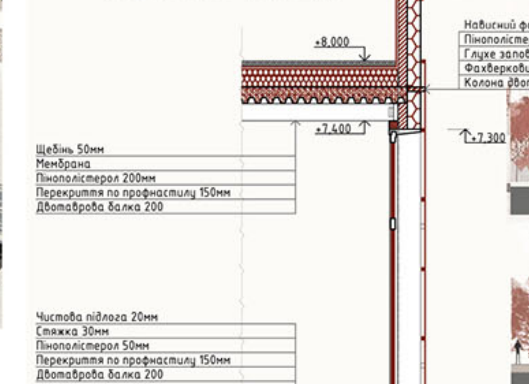
Розріз по стіні (М 1:20)
