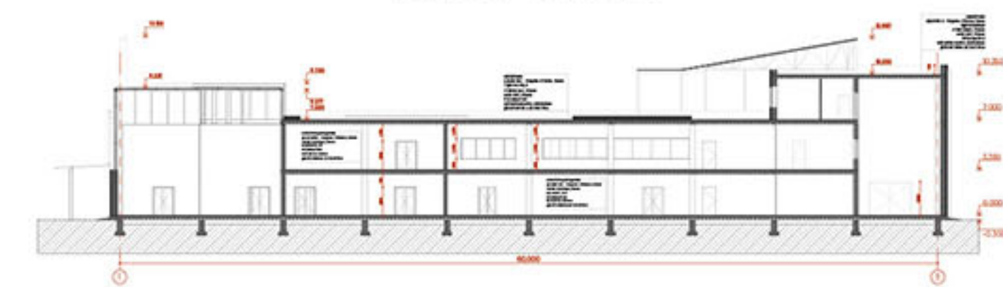
Розріз 2-2 М1:200
