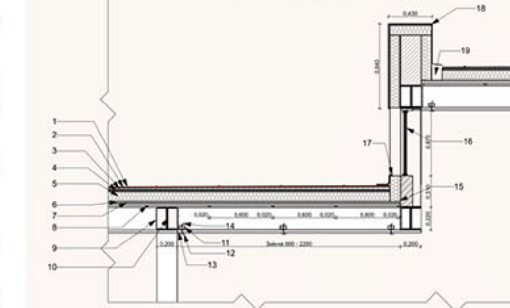
Вузол будівлі Б (М 1:20)
