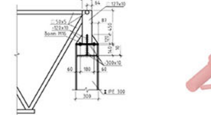
Вузол Б
