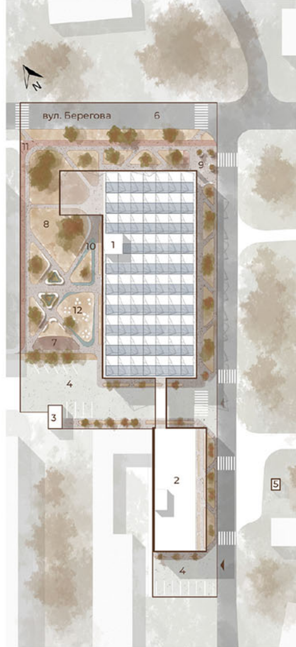
СХЕМА ГЕНЕРАЛЬНОГО ПЛАНУ М 1:200
