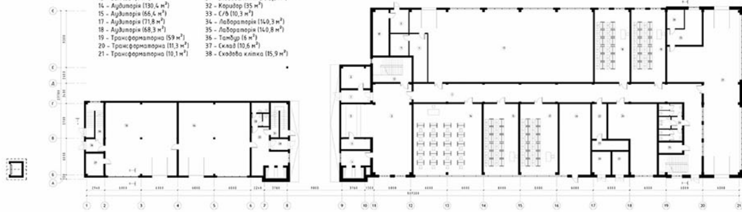
ПЛАН ПОВЕРХУ НА ВІДМ. +0.000 М 1:100
