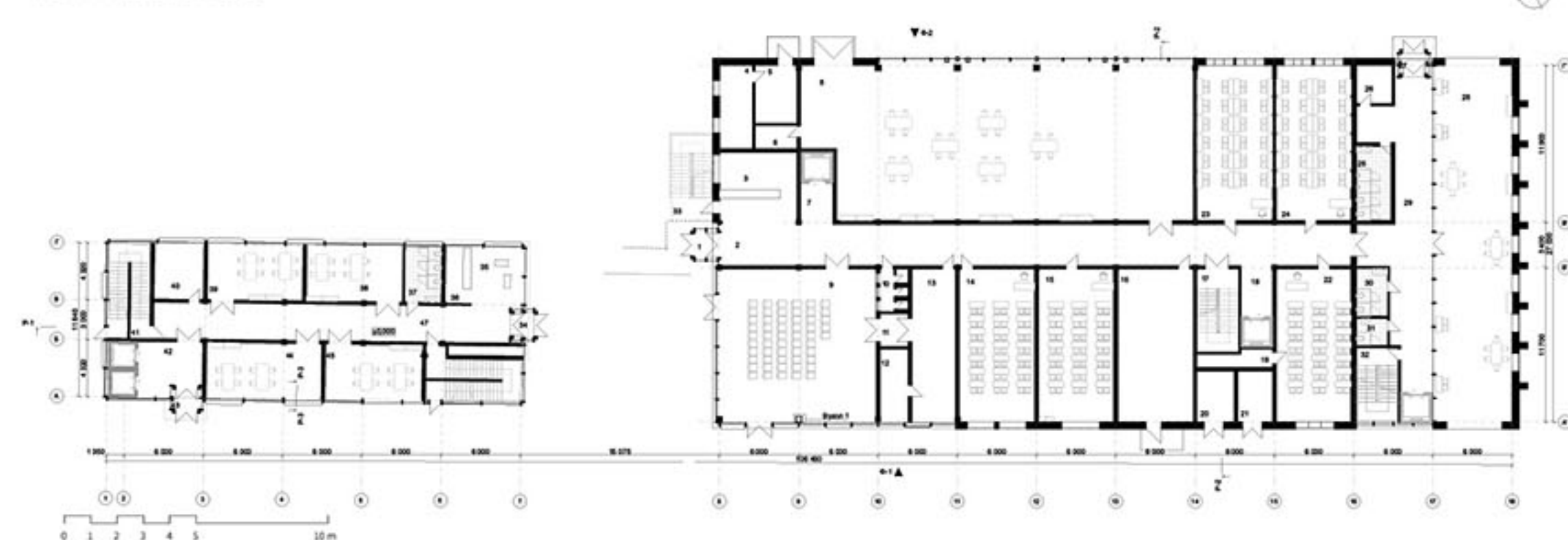
ПЛАН 2 ПОВЕРХУ М 1:200
