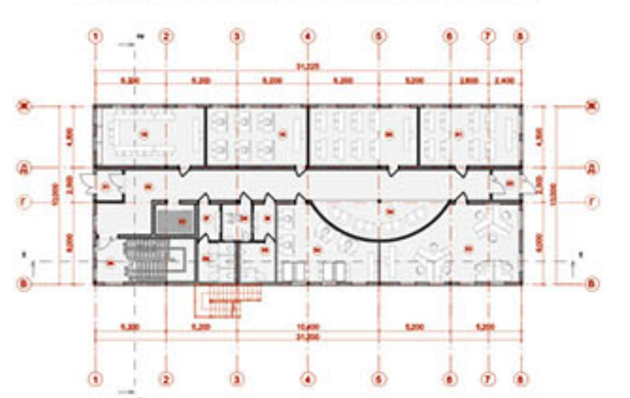
План на відмітці ±0,000 М1:200
