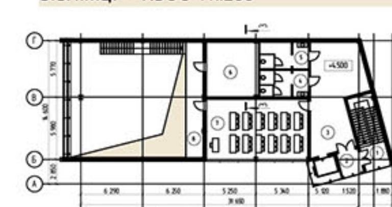
План другого поверху корпусу №11 на відмітці +4.500 М1:200
