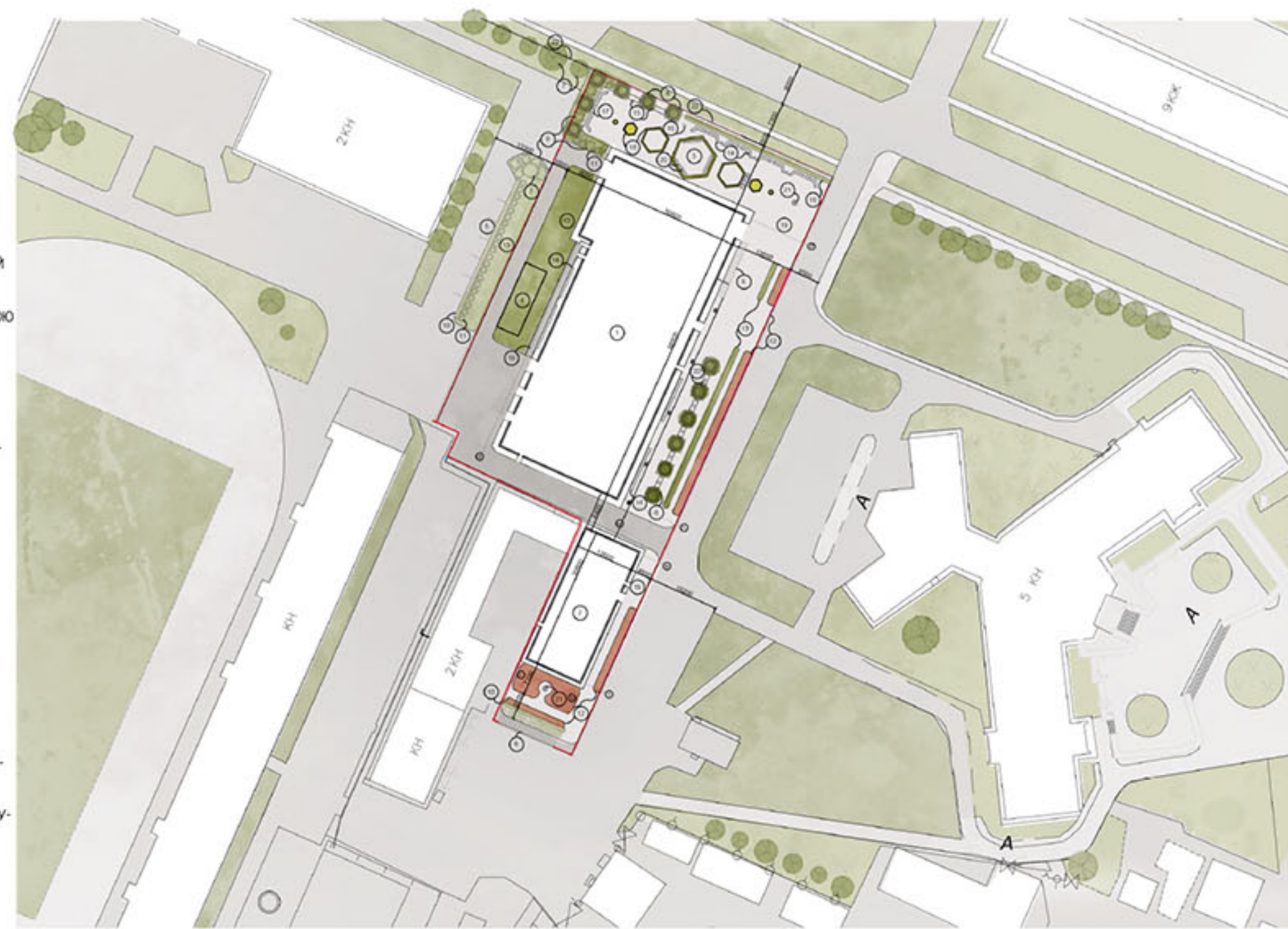
СИТУАЦІЙНА СХЕМА, М 1:20 000 ГЕНПЛАН, М 1:500
