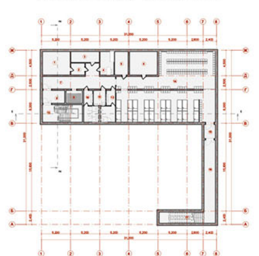
План на відмітці -3,000 М1:200
