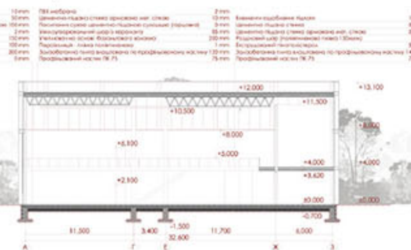
Розріз 2-2 М 1:200
