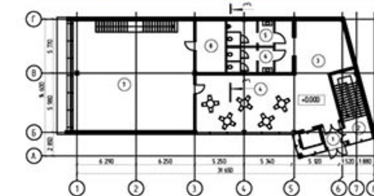
План першого поверху корпусу №11 на відмітці +0.000 М1:200
