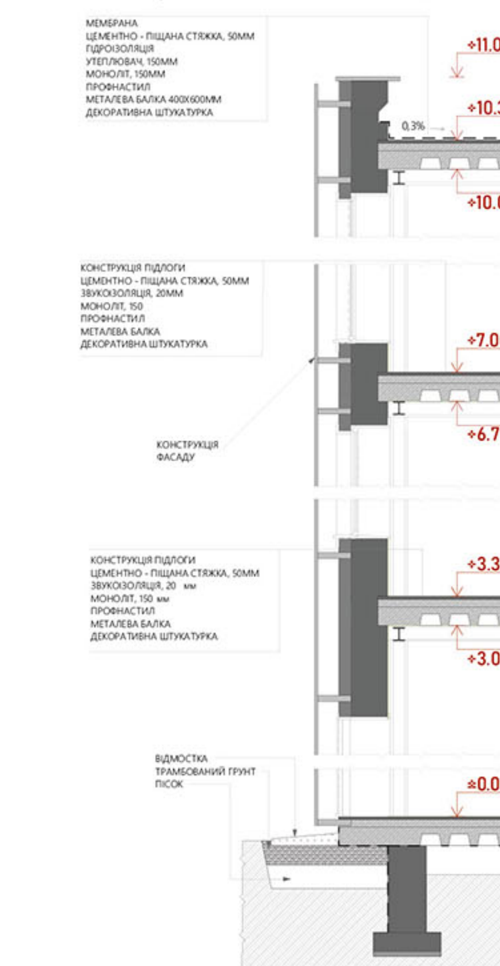
Розріз детальний по стіні(3-3) М1:20
