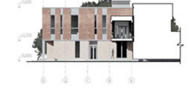
Фасад в осях Е-Б М 1:200
