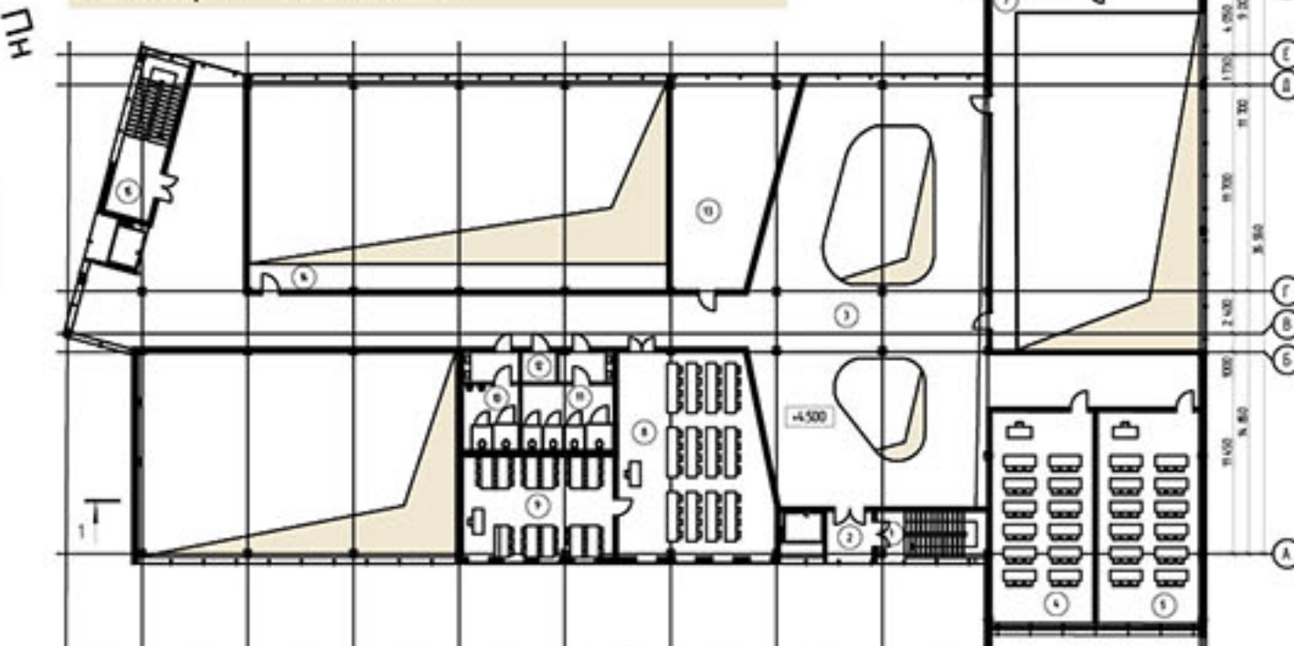
План другого поверху корпусу №7 на відмітці +4.500 М1:200
