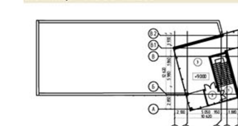
План третього поверху корпусу №11 на відмітці +9.000 М1:200
