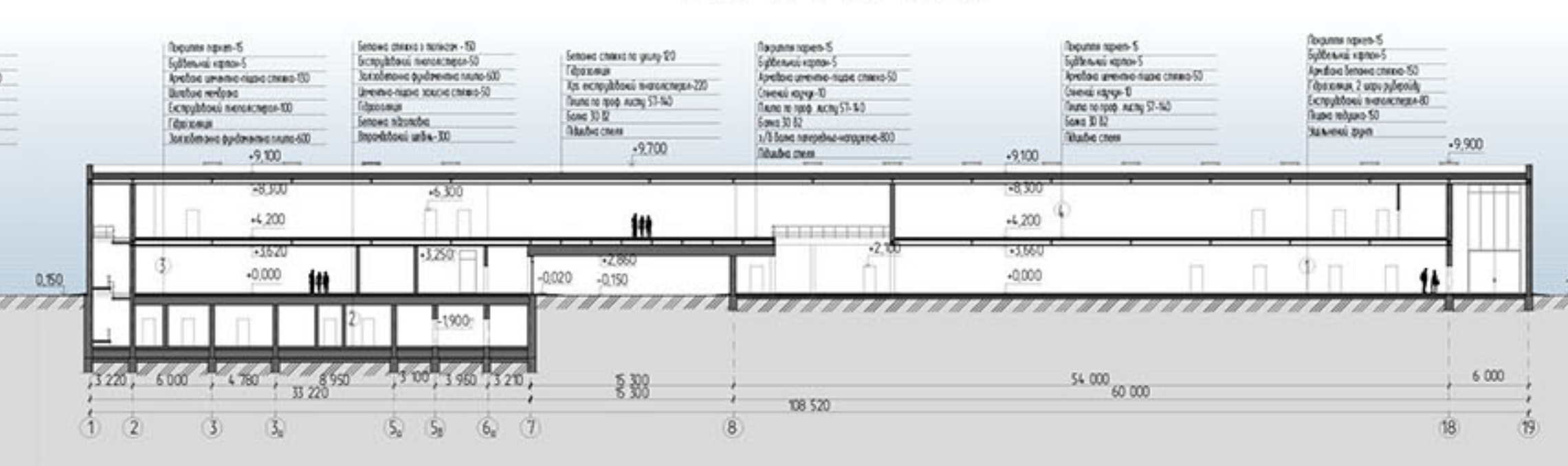
Розріз 1-1 М 1:200
