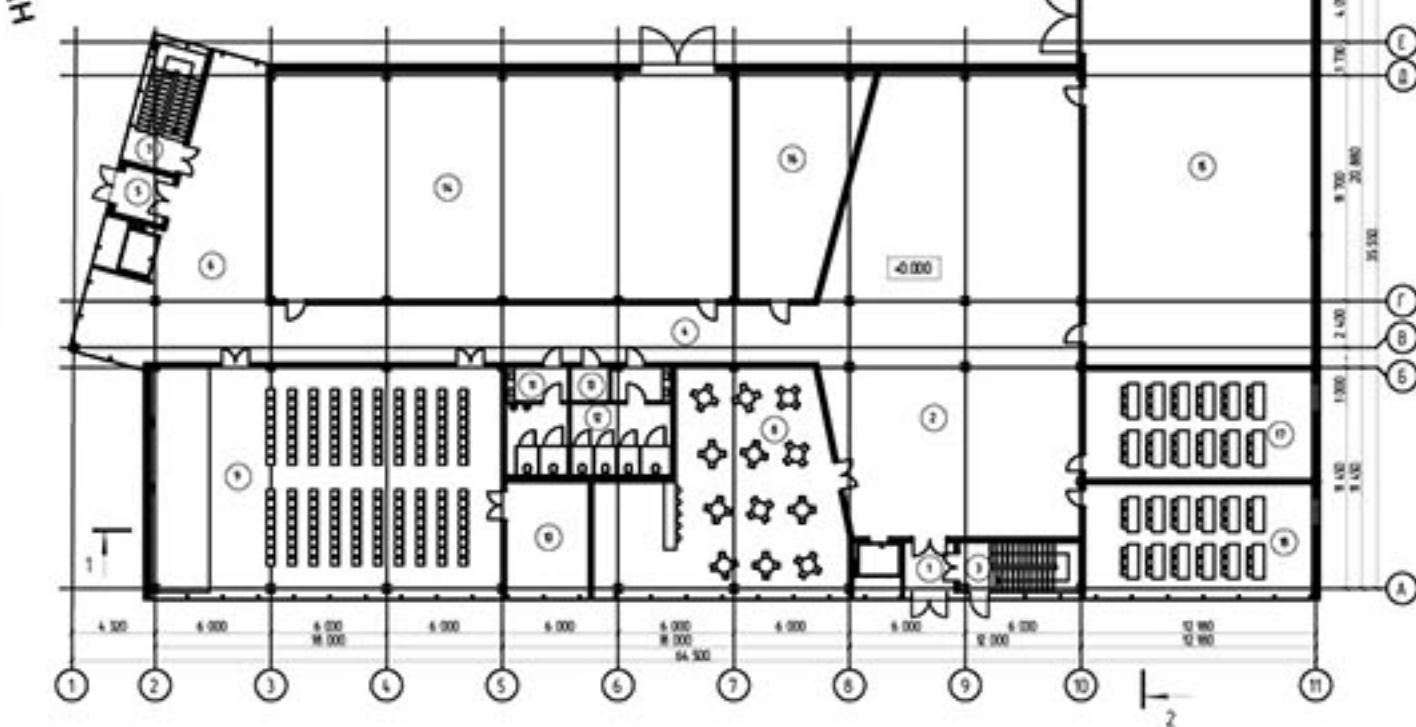
План першого поверху корпусу №7 на відмітці +0.000 М1:200
