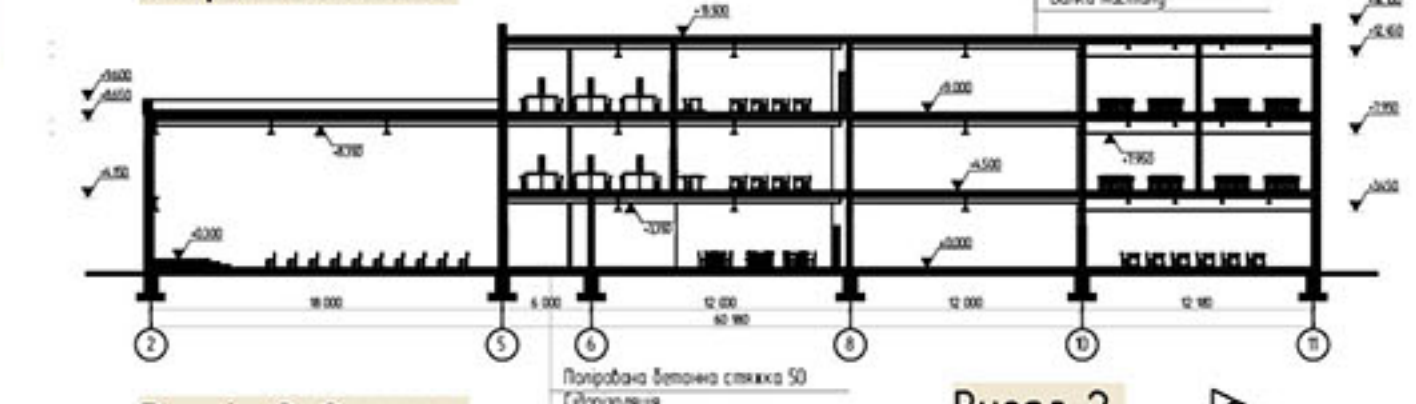
Розріз 2-2 М1:200
