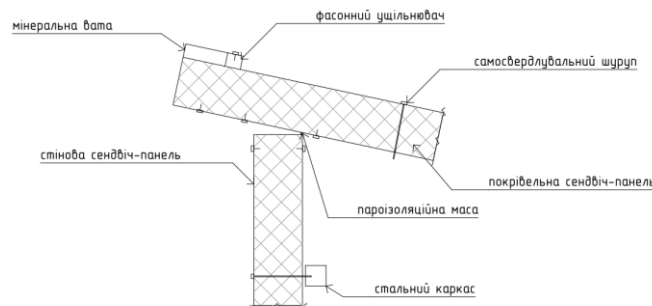
Вузол Б
