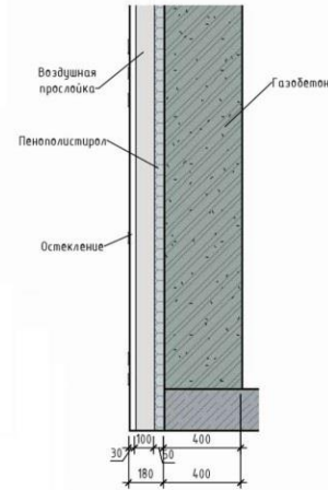
Розріз по стіні М 1:20 Влаштування вентиляційного фасаду
